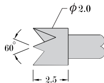
QSP-11F
