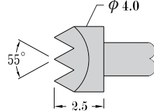
QSP-11H
