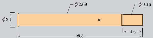
QSR-11V1
