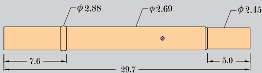
QSR-11W1
