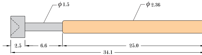
QSP-11B
